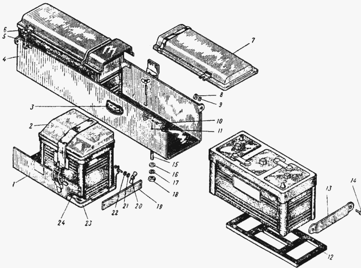
Рис. 48. Установка аккумуляторных батарей
